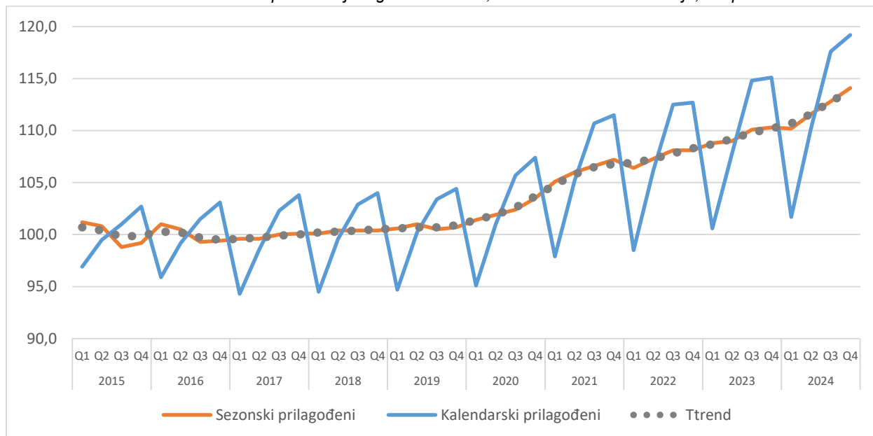
Grafikon 9: Indeksi proizvodnje u građevinarstvu, kvartalne vremenske serije, ukupno
